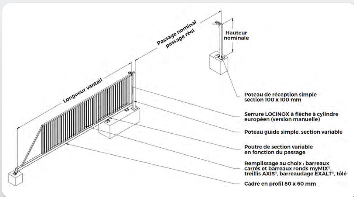
Poutre 150x120 mm pour les passages de 3 m à 8 m
