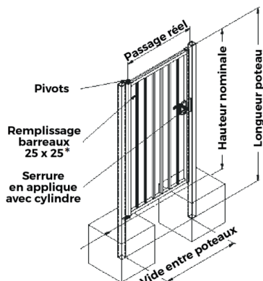
Portillon 1 vantail
